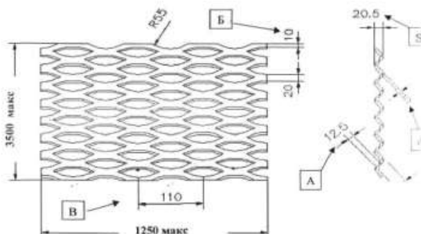
Основные параметры и размеры стальных просечно-вытяжных листов
